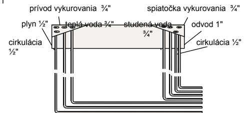
prívodné potrubia sprava
