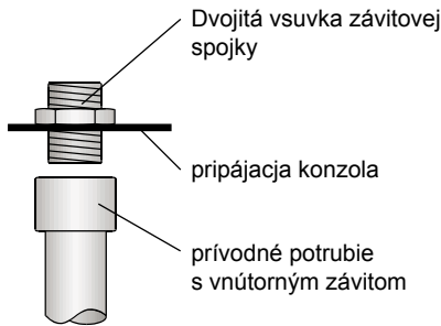
dvojitá vsuvka na pripájacej konzole
