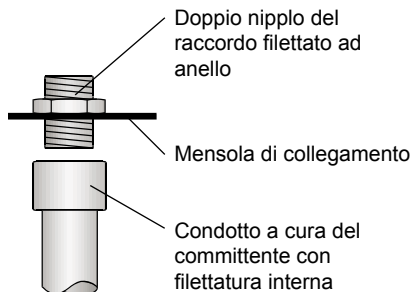
Doppio nipplo su mensola di attacco
