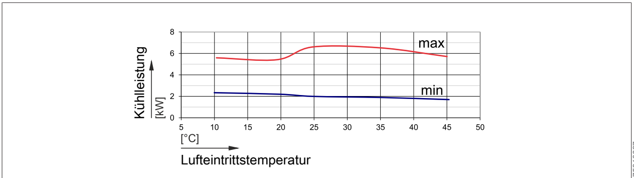
Abb. 17: Kühlleistung CHA-0 bei einem Vorlauf von 7 °C
