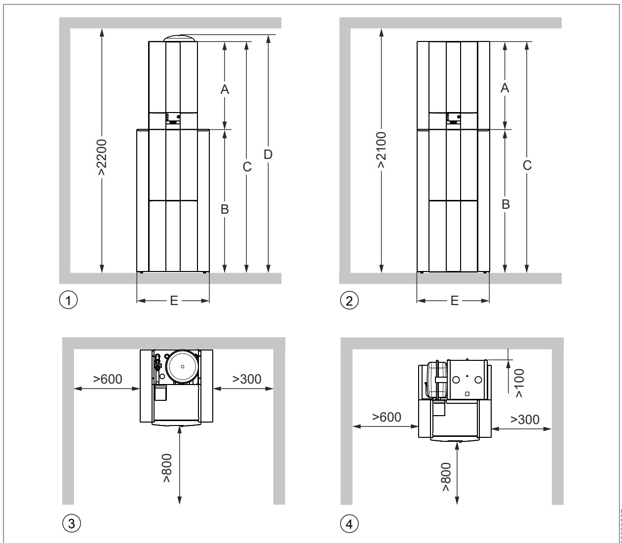
① Vorderansicht CHC-Monoblock / 200
