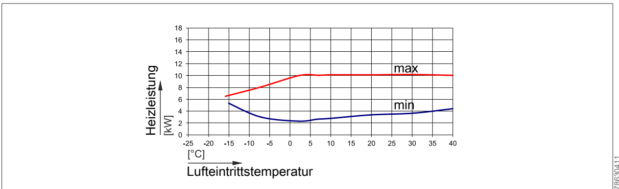
Abb. 15: Heizleistung CHA-10 bei einem Vorlauf von 65 °C
