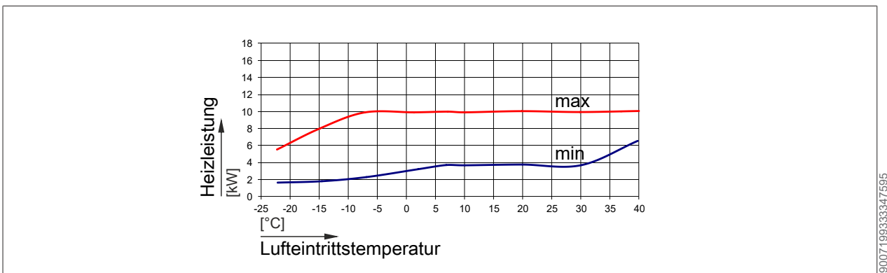
Abb. 11: Heizleistung CHA-10 bei einem Vorlauf von 25 °C
