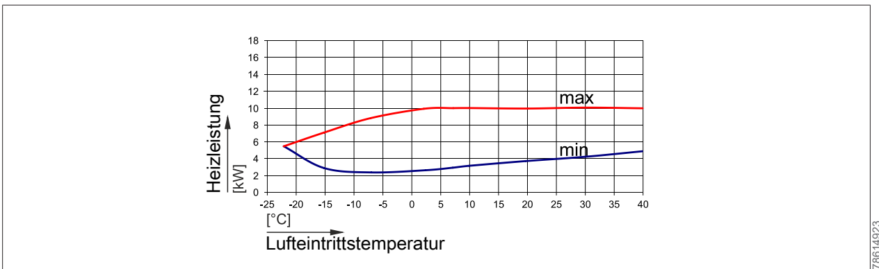
Abb. 14: Heizleistung CHA-10 bei einem Vorlauf von 55 °C
