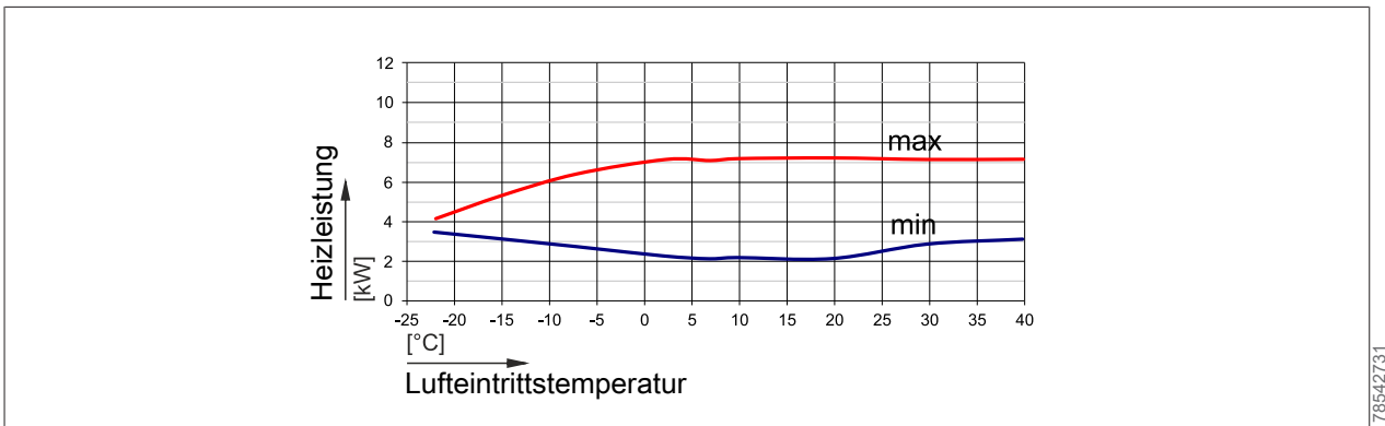
Abb. 9: Heizleistung CHA-07 bei einem Vorlauf von 55 °C
