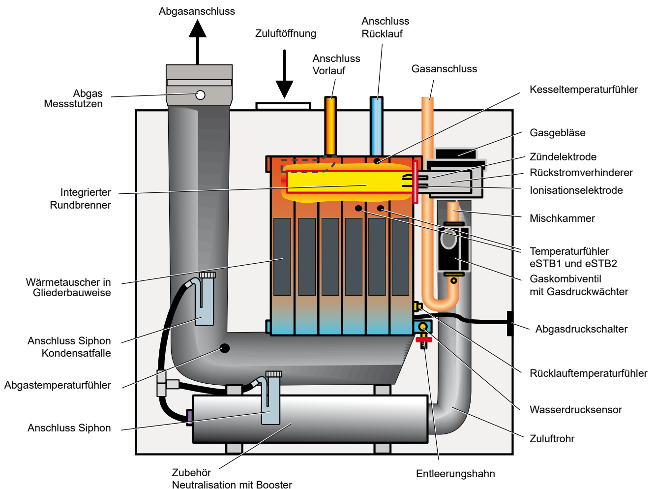
Aufbauschema MGK-2
