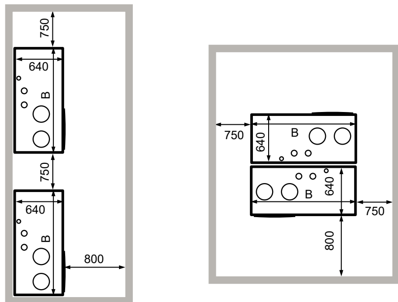
Bild: 2 - 4 Kessel im Heizraum, nebeneinander
