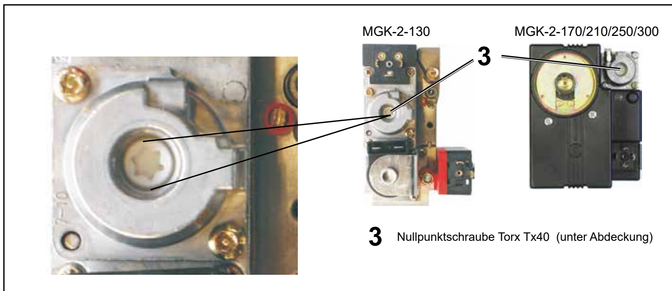
Bild: Gaskombiventil
