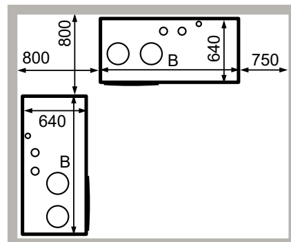
2 Kessel im Heizraum
