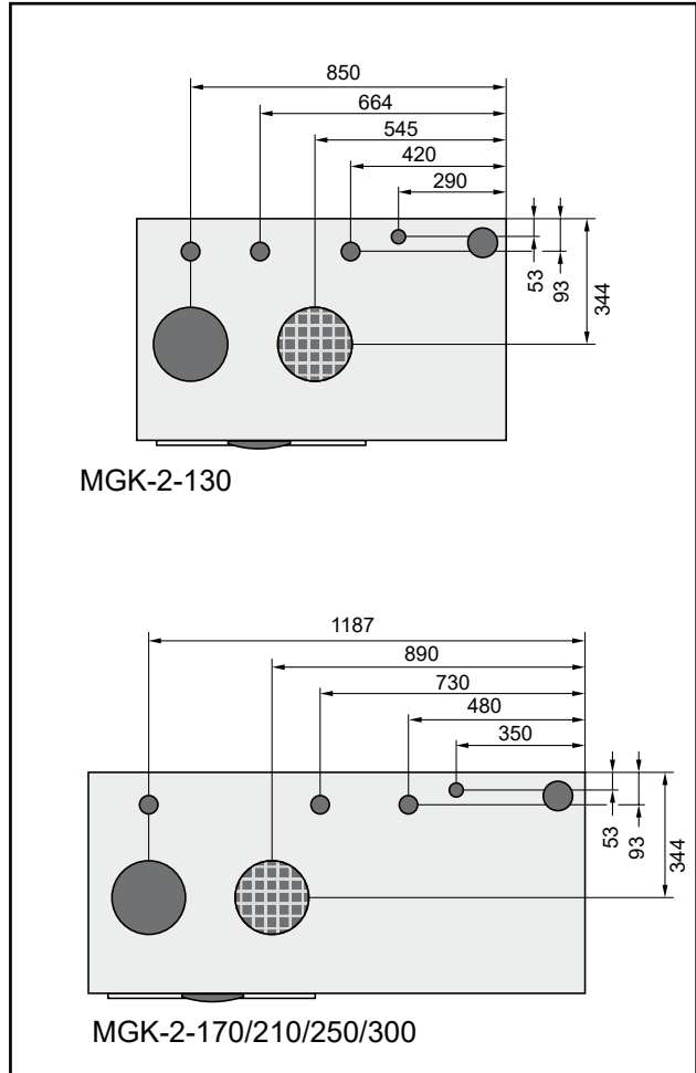
Bild: Anschlussmaße
