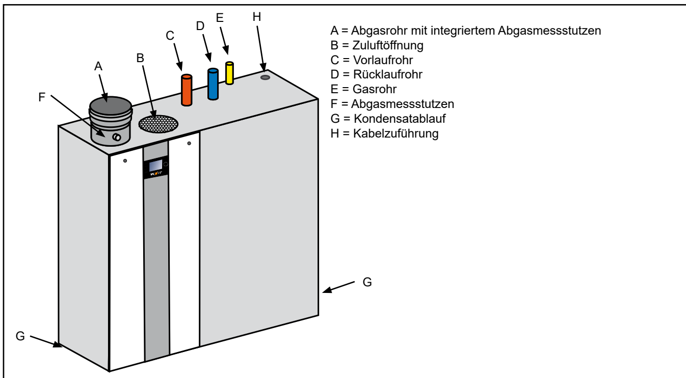
Bild: Anschlüsse
