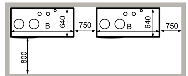
2 - 4 Kessel im Heizraum, nebeneinander
