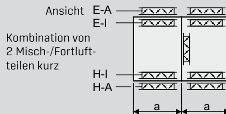
Baugröße Abmessungen (LxBxH)
