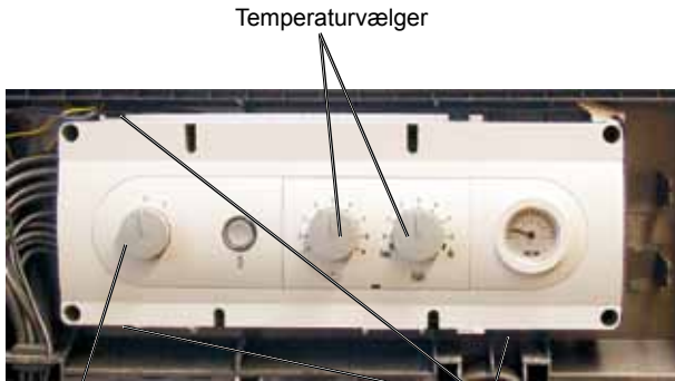
Indkoblingskontakt ON/OFF
