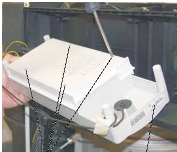
Viti coperchio parete posteriore Adesivo „Mat-No.“
