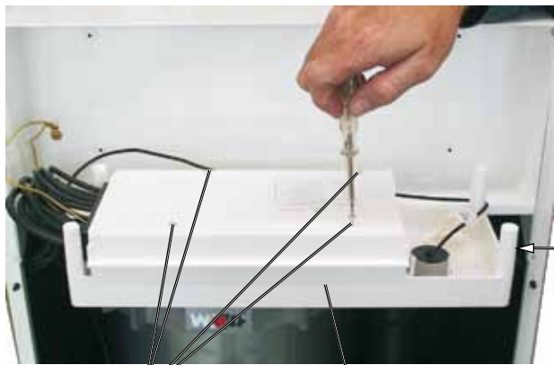
Vis du couvercle de la paroi arrière
