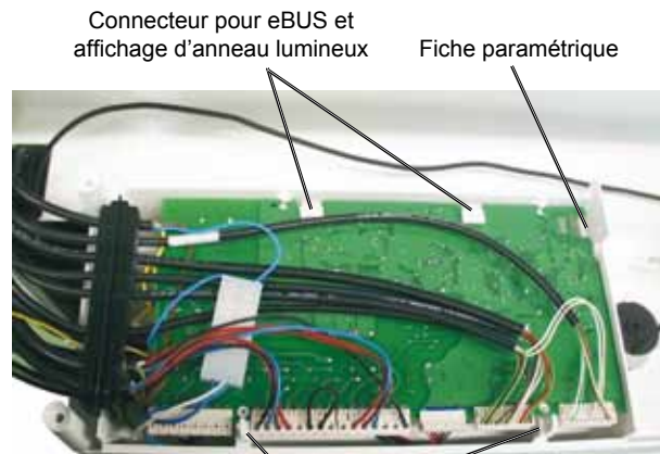
Clips d'arrêt servant à la fixation du circuit imprimé
